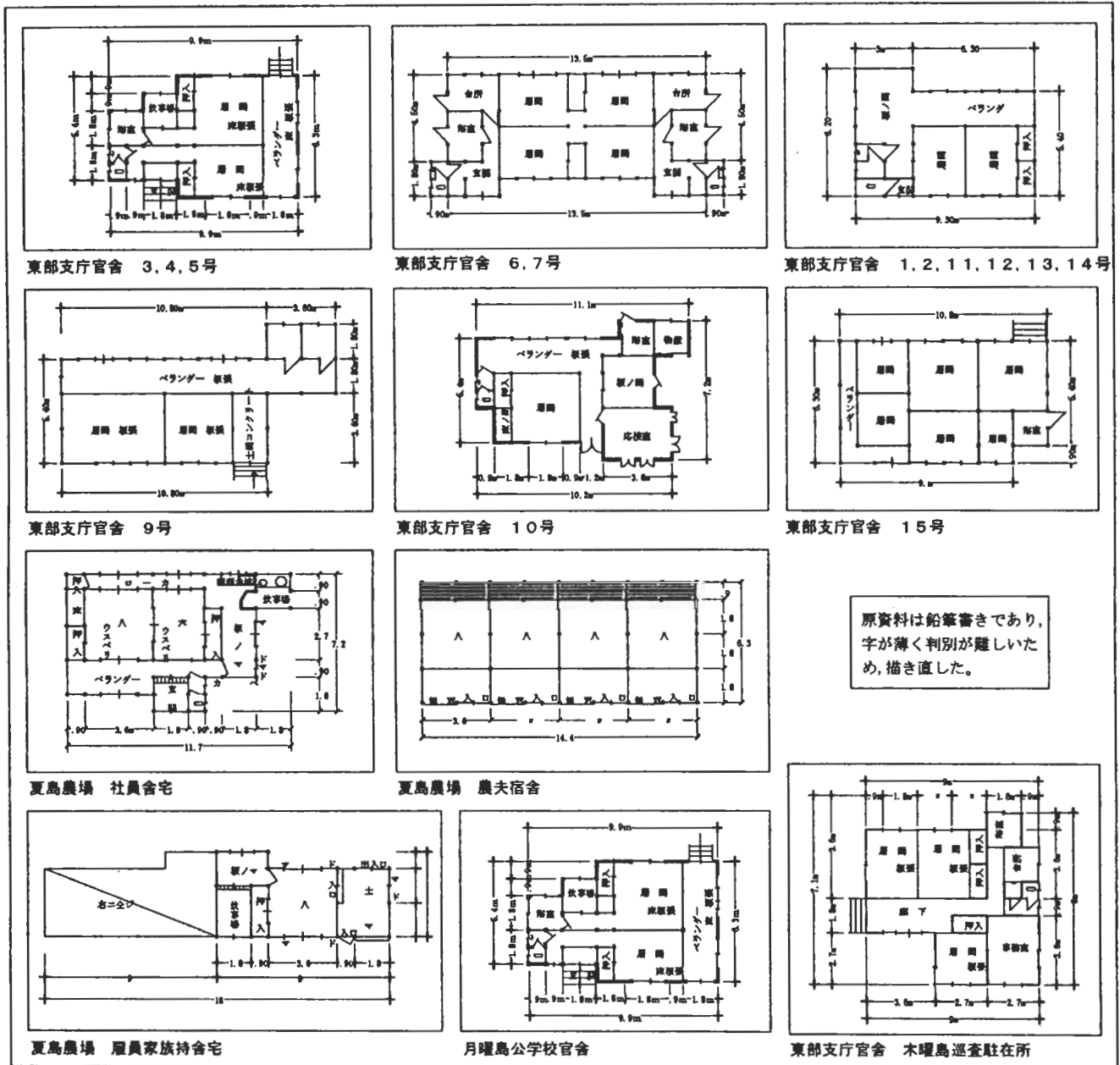
図1 『南洋庁東部支庁関係書類』に含まれる官舎と社宅の図面（一部）
