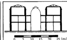
図8 パリ内部測定地点断面図
