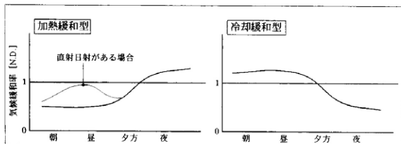
図15 半戶外空間の気候緩和率の一日のうちの变化の様子
