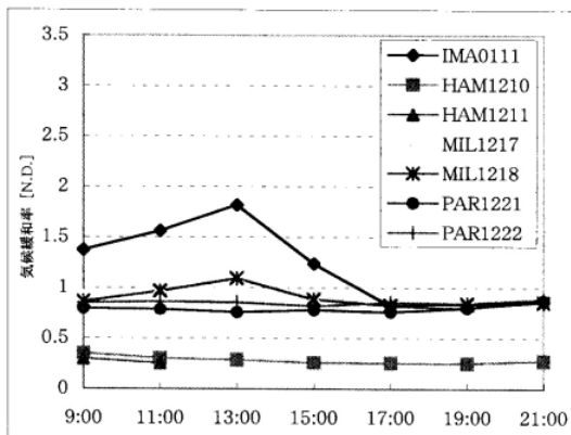
図21 各地の冷却緩和型半戶外空間(冬季)の気候緩和率
