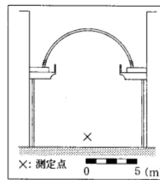
図16 今治の断面図
