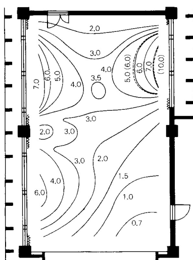
図1 昼光率分布の例（出典：参考文献 [3]，p. 74）
