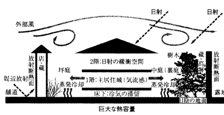
植栽や水面を有して低温面を形成する二つの中庭の空間ボリュームの違いによって生じる圧力差を利用し、室内に風を発生させ、深い軒庇、蔵や高層によって日射を遮蔽している京都の町家。 03
