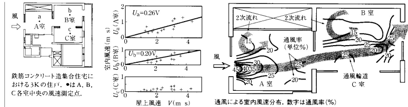
鉄筋コンクリート造集合住宅における3Kの住戸。●はA, B, C各室中央の風速測定点。 屋上風速 V と室内風速 U の関係 風は風上開口と風下開口を結ぶ線に沿って通風輸道を生じる。そこでの風速は外部の風速に比例し、通風率(=室内風速/外部風速)は一定となる。しかし、間仕切り開口で接する他の通風輸道から生ずる室の風速は、外部の風速に関係なく非常に弱い。通風時の風速分布は複雑であり、通風輸道の風は同じ室内の隣接空間に2次気流を派生させる。
