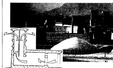
日射が塔が熱せられ、室内の暖かい空気が上昇し、涼しい空気が引き込まれる。高温乾燥地域で換気塔を備え、家の中に風道を作っている例。
