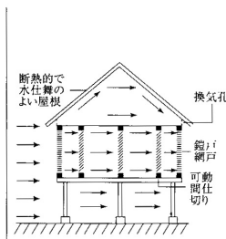
高温多湿地域の開放的な住居。風上と風下で大きな開口を設ける。
