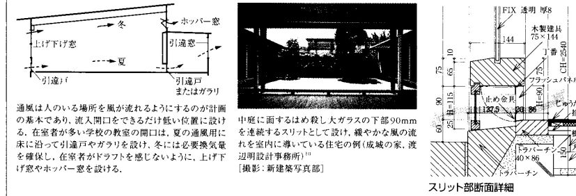
通風は人のいる場所を風が流れるようにするのが計画の基本であり、流入開口をできるだけ低い位置に設ける。在室者が多い学校の教室の開口は、夏の通風用に床に沿って引違戸やガラリを設け、冬には必要換気量を確保し、在室者がドラフトを感じないように、上げ下げ窓やホッパー窓を設ける。 中庭に面するはめ殺し大ガラスの下部90mmを連続するスリットとして設け、緩やかな風の流を室内に導いている住宅の例(成城の家、渡辺明設計事務所) [撮影: 新建築写真部] スリット部断面詳細
