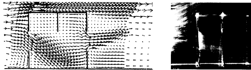
通風の効果は室内の風速分布によっては決定される。間仕切りを有する独立模型内の通風時風速の断面内分布に、乱流数値シミュレーションによる風速ベクトル分布と風洞模型実験により可視化したものを比較すると、両者の気流パターンはよく一致している。
