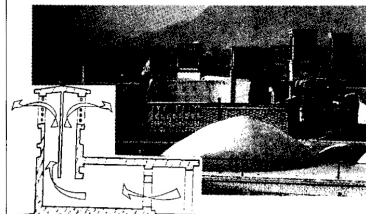
高温多湿地域の開放的な住居。風上と風下に大きな開口を設ける。
