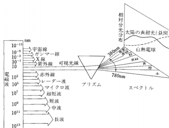
図 電磁波の中の可視光（出典：参考文献 [ 1 ]）
