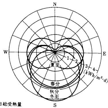
図9-5 東京における季節ごとの各方位に入射する日射量 1)
