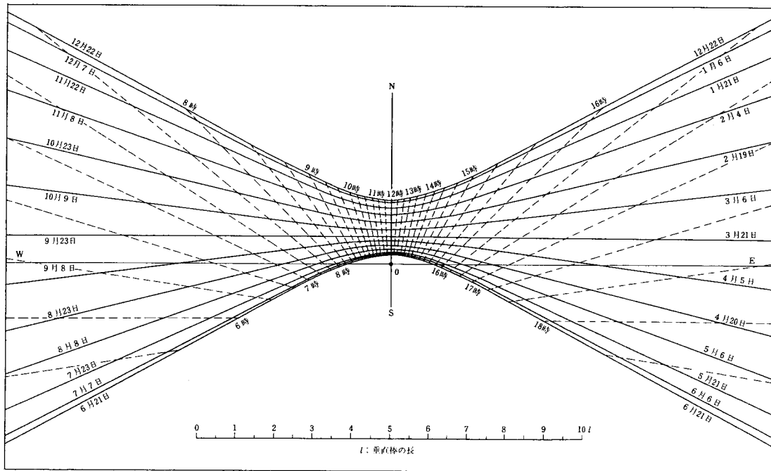
図8-2 水平面日影曲線図（北緯35°）
